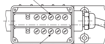
Amplitudenanpassung SLAVE-Stellmagnet
