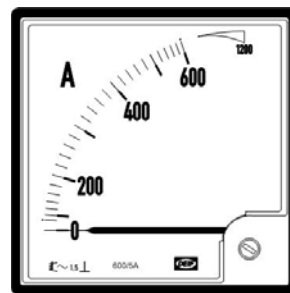
EQ96-x (ammeter)
