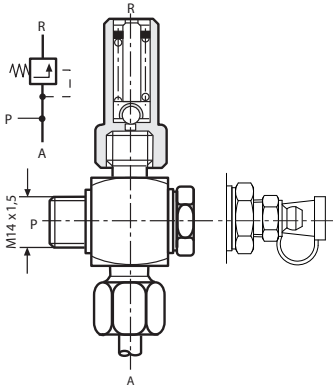
Druckbegrenzungsventil, Abb. 2
