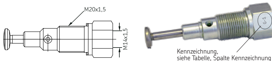
zwangsgeführte Pumpenelemente G-1 ohne Druckbegrenzungsventil, Abb. 8
