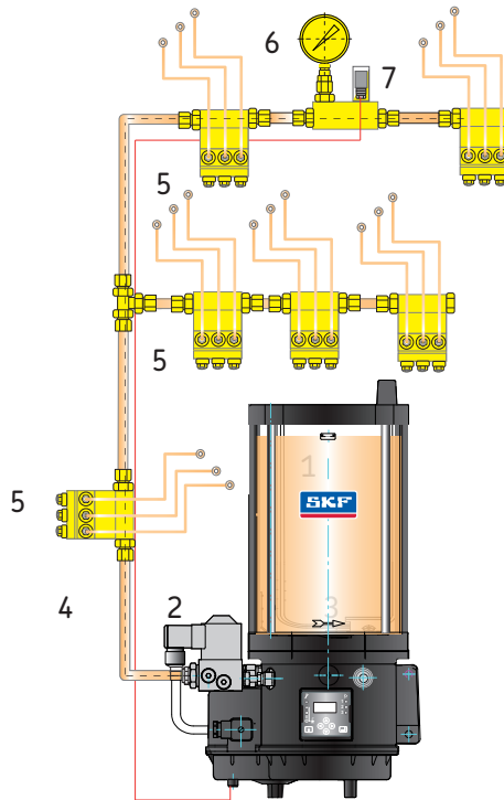
Beispiel einer Einleitungsanlage mit KFGL-Pumpenaggregat, Abb. 8
