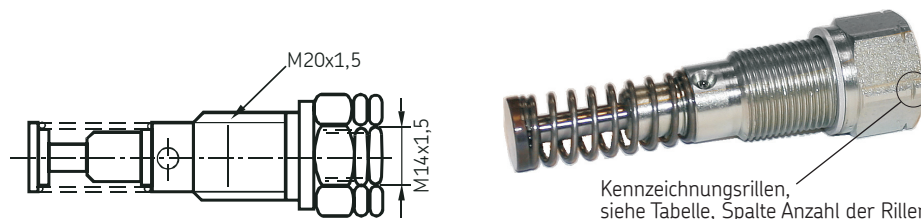
federrückgeführtes Pumpenelemente KFG1.U1 ohne Druckbegrenzungsventil, Abb. 6
