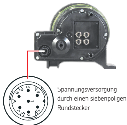
KFGL Spannungsversorgung, Abb. 22
