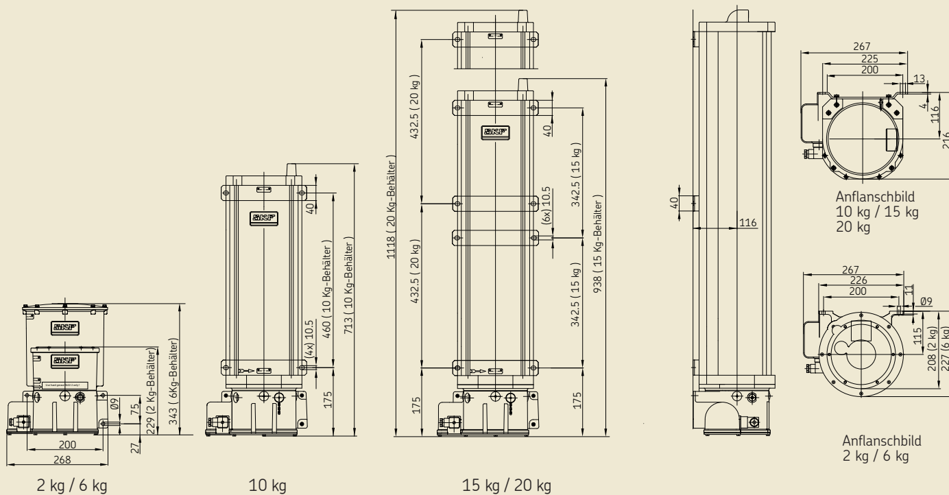
Montagemaße, Abb. 2
