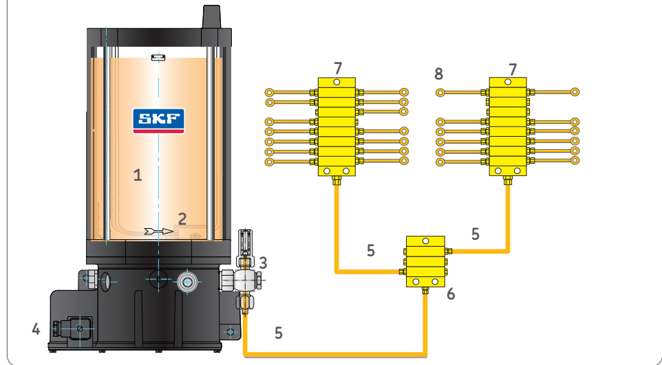
Progressivanlage mit KFG-Pumpenaggregat
