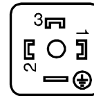
Bild 9. Steckverbinder X1 Steckverbinder nach DIN 175301-803
