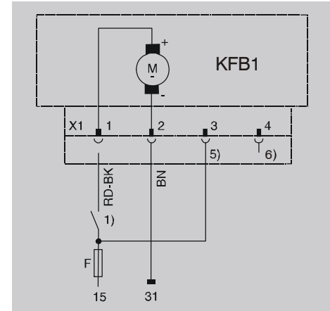
Bild 4. Elektrischer Anschluss KFB1 15 + Potential Versorgungsspannung 31 - Potential Versorgungsspannung 1) Externes Steuergerät; Relaiskontakt „Pumpe EIN“ 5) Anschluss Drucktaster für Zwischenschmierung 6) PIN ohne interne Verbindung F Sicherung
