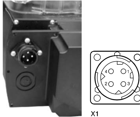
Bild 3. Rundsteckverbinder X1 nach DIN72585-A1-4.1-Ag/K1
