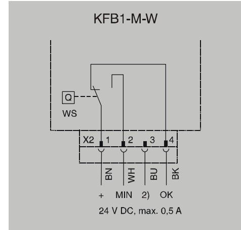
Bild 13. Anschluss Füllstandsüberwachung KFB1-M-W
