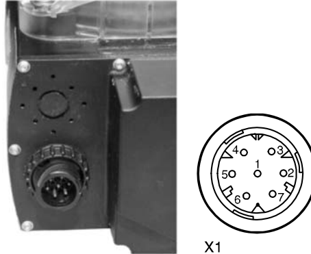
Bild 7. Rundsteckverbinder X1
