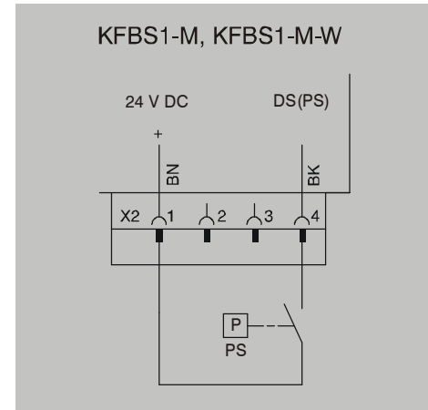
Bild 16. Elektrischer Anschluss X2 KFBS1-M und KFBS1-M-W PS Druckschalter
