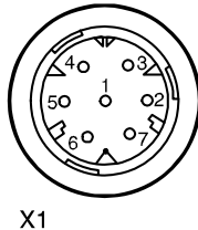
Bild 6. Elektrischer Anschluss KFB1-W
