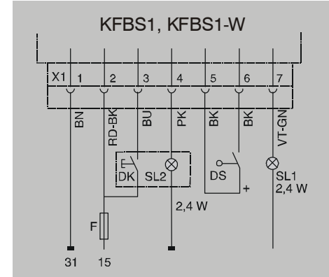
Bild 8. Elektrischer Anschluss KFBS1 und KFBS1-W
