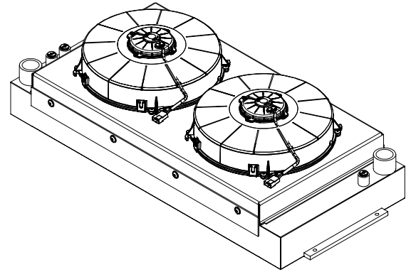
Kühlpaket sowie Gehäuse ähnlich RAL 9005 Cooling block and housing similar to RAL 9005
