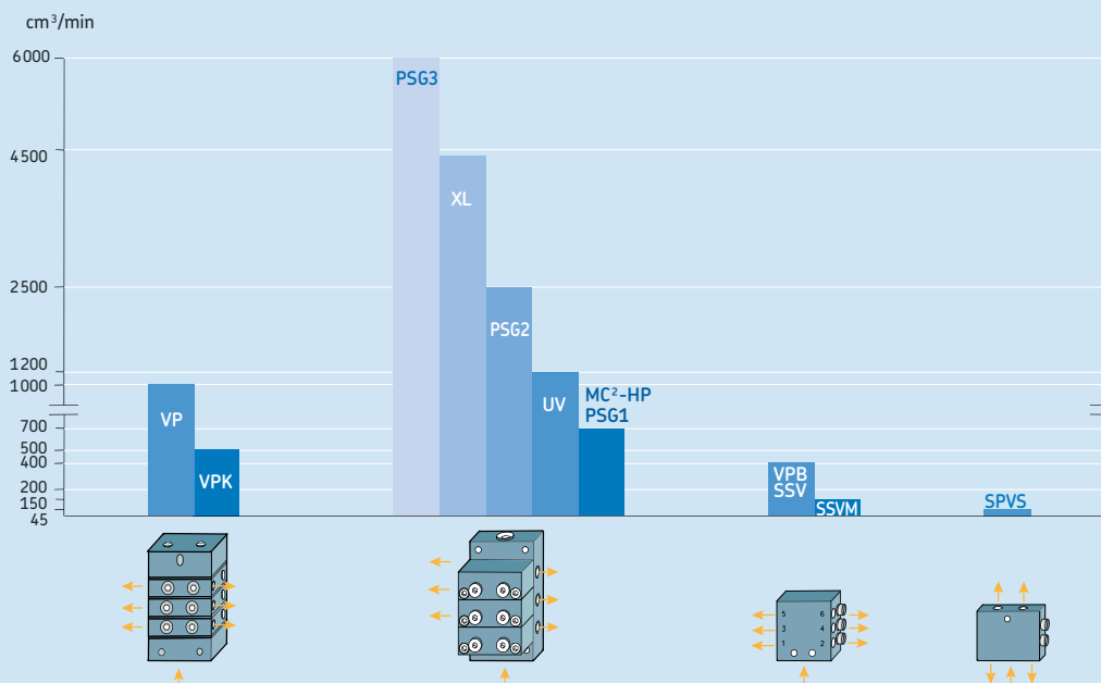
Übersicht SKF Progressivverteiler, Einlassvolumenstrom
